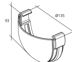
Заглушка желоба ПВХ 135/90
