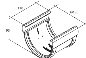
Соединитель желоба ПВХ 135/90
