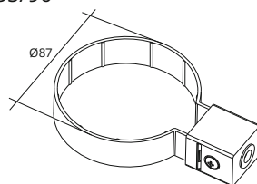
Хомут трубы Klicker ПВХ Premium 135/90
