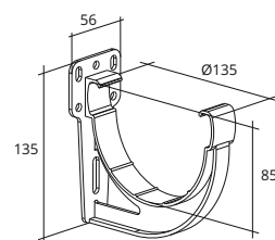
Кронштейн желоба ПВХ 135/90
