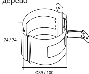
Металлический хомут трубы на дерево
