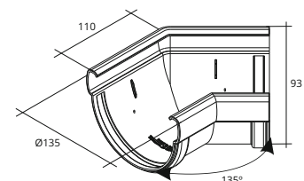
Угол желоба 135° ПВХ 135/90
